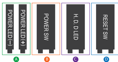
前面板导线
